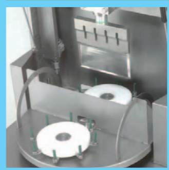
Machine à trancher pour produits circulaires
